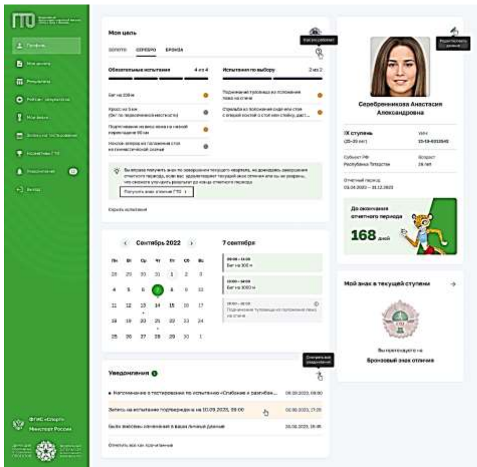
Рисунок 25. Страница «Профиль»
