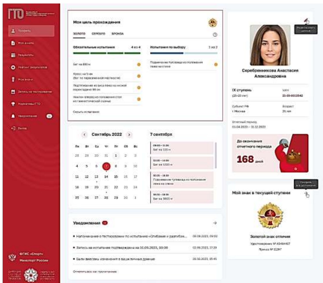
Рисунок 24. Страница «Профиль»
